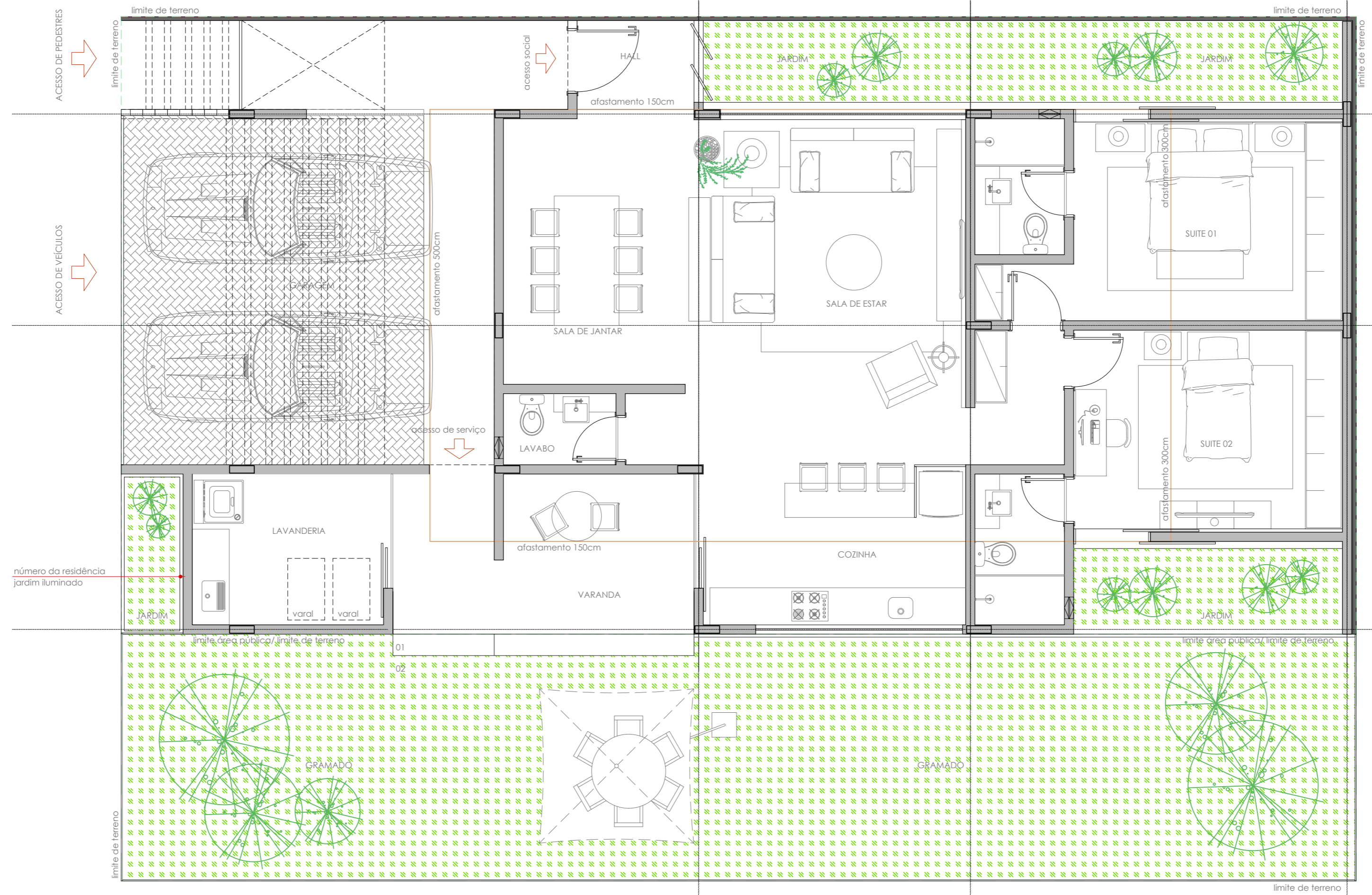
PLANTA BAIXA: Pavimento Térreo escala 1:75
